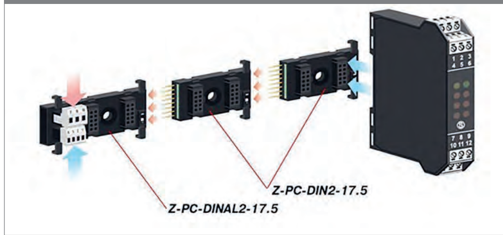
ESEMPIO DI COLLEGAMENTO PER MODULI DIN 17.5 mm
