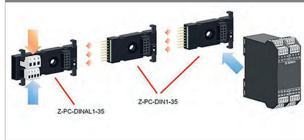
ESEMPIO DI COLLEGAMENTO PER MODULI DIN 35 mm
